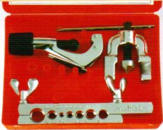
CT-1226 ชุดบานพับ ชั้นเดียวพร้อมตัด (3/16"-5/8")
